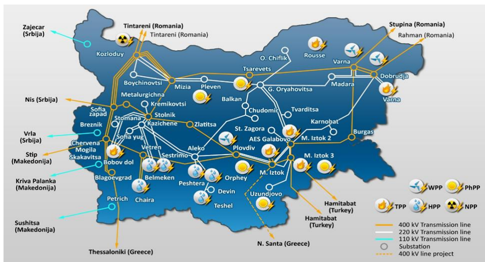
Фигура 60: Карта на преносната инфраструктура ВН
