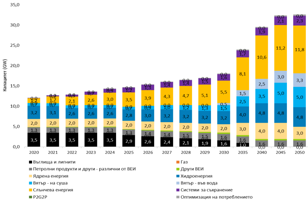
Графика. 14 Инсталирани производствени мощности по вид гориво до 2050 г., GW
