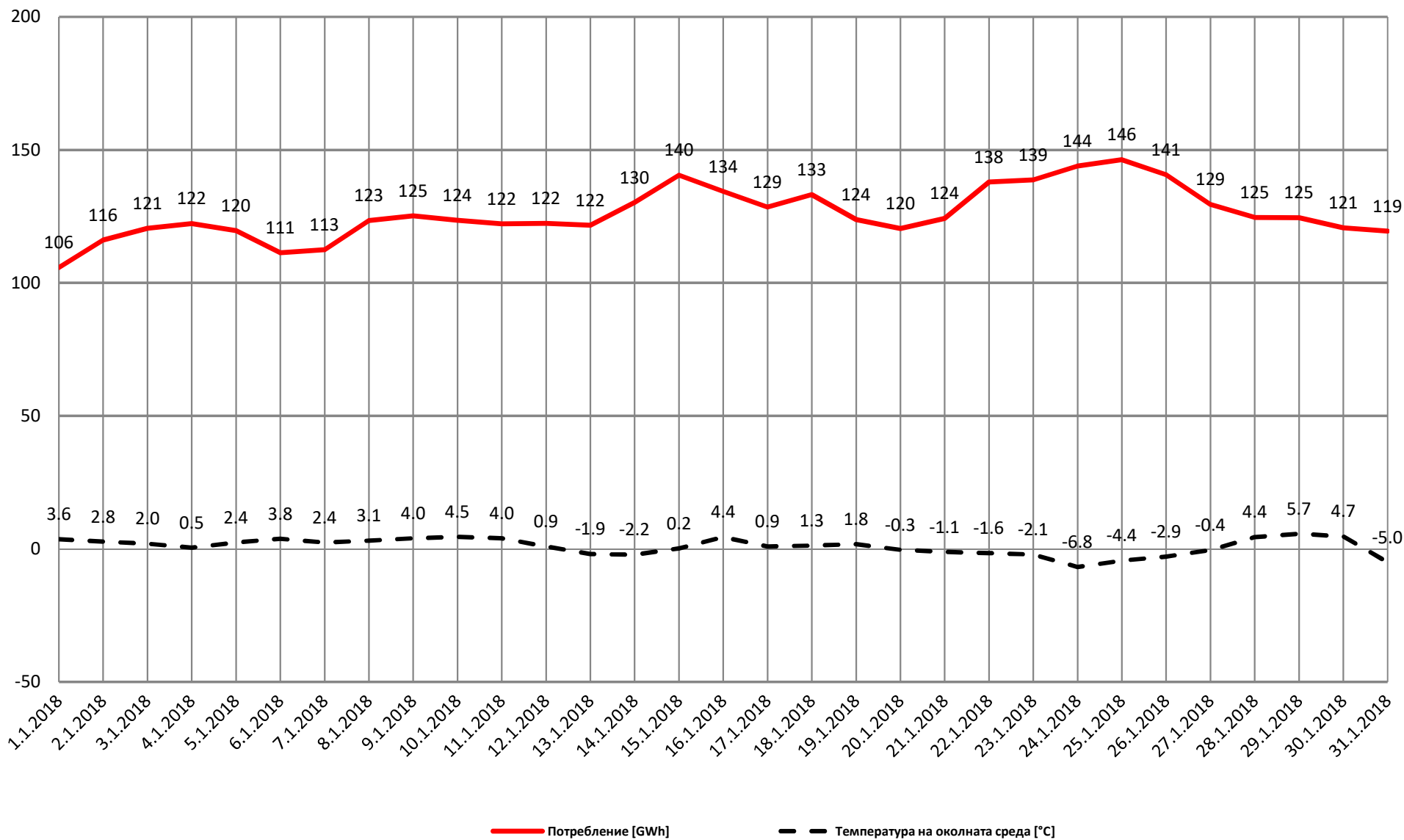
Приложение 5.2 - Съпоставяне потреблението на газ в България и околната температура (гр. София) за януари 2018 г.
